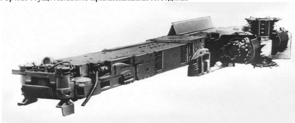
Рис. 1 – Комбайн типа УКР-1
